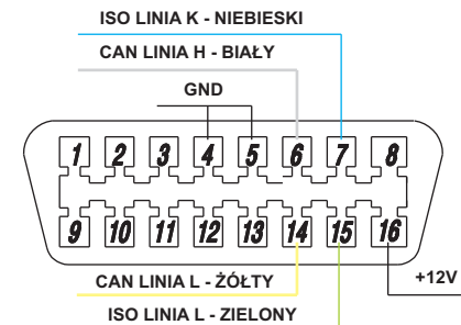
WIDOK OD CZOŁA OBUDWY
